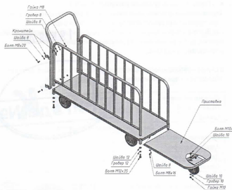
Схема сборки тележки
